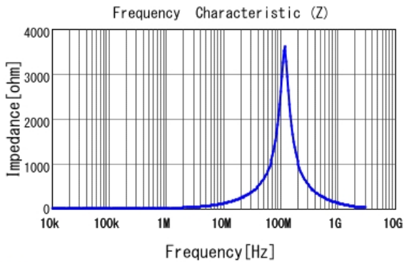
■ 1227AS-H-2R2M |Z|
