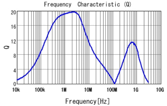
■ 1227AS-H-2R2M Q
