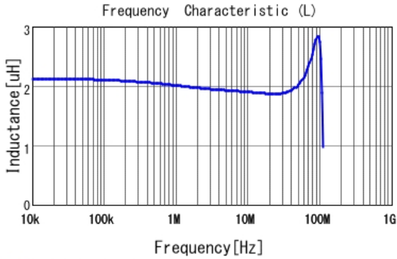
■ 1227AS-H-2R2M L
